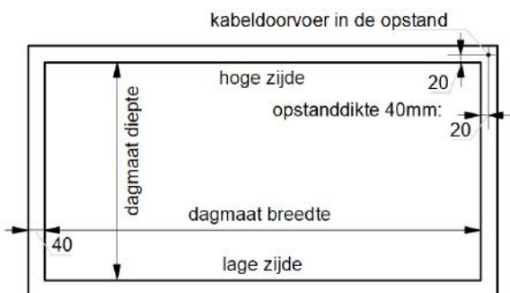
Maatvoering kabeldoorvoer in de opstand bij 40mm opstanddikte
