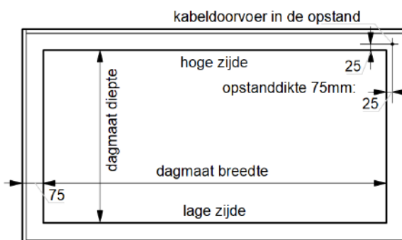
Maatvoering kabeldoorvoer in de opstand bij 75mm opstanddikte DL75
